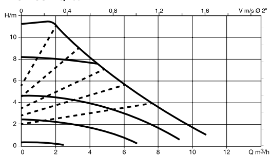
EVOPLUS 110/180 XM
